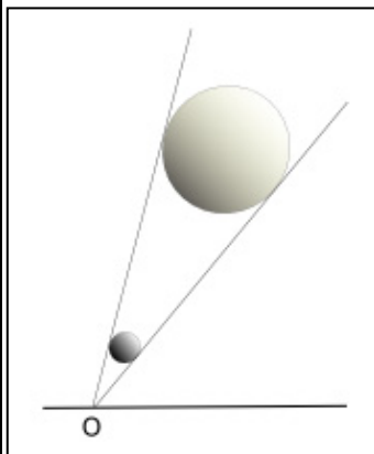
Modelo en el que dos cuerpos, tendrían el mismo tamaño aparente.
